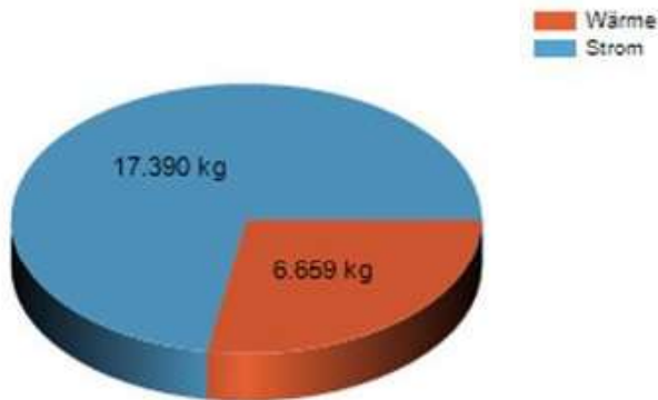
CO 2 -Emissionen
