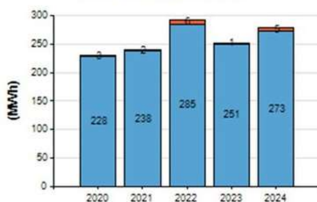
Gesamtenergieverbrauch
