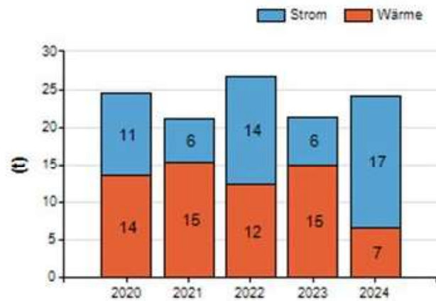
CO 2 -Emissionen
